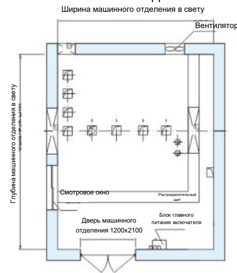
Горизонтальная проекция машинного отделения
