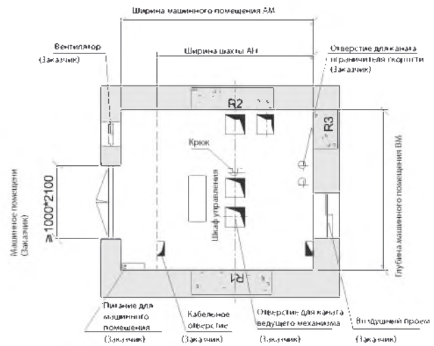
Схематический чертеж зарезервированного машинного помещения
