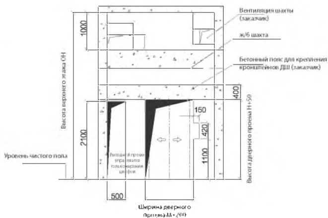
План шахты
