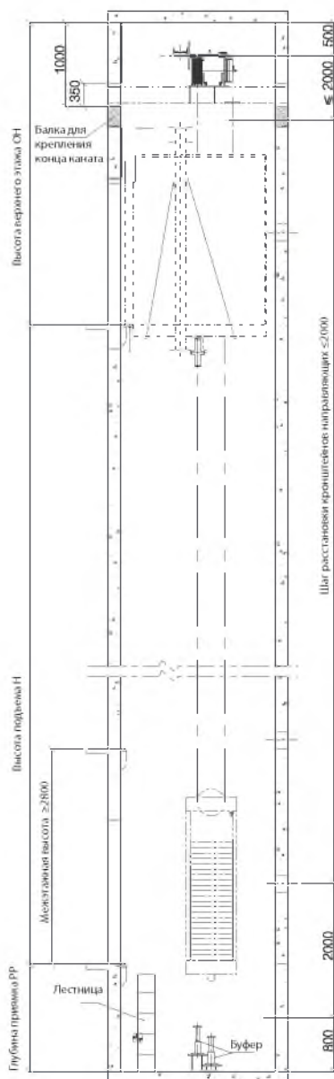
Вертикальный разрез шахты
