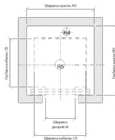
План шахты
