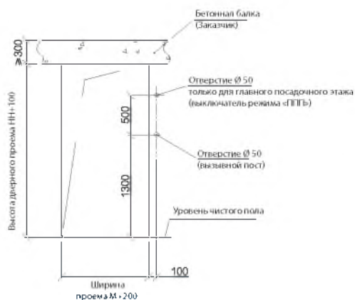
Дверной проем. Вид с этажной площадки
