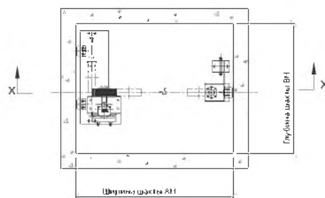
План шахты (оборудование в оголовке)
