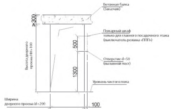
Дверной проем. Вид с эстажной площадки
