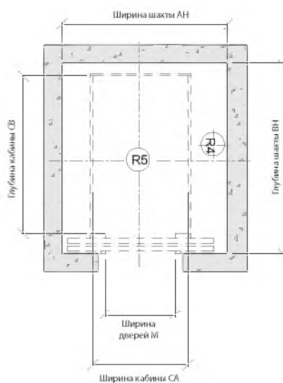
План шахты
