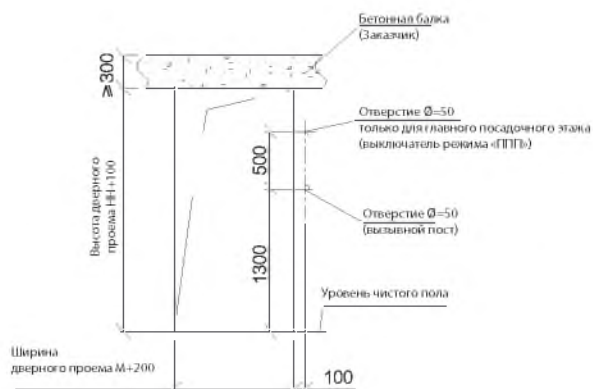
Дверной проем. Вид с этажной площадки
